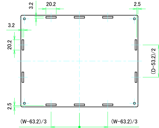
上カバー裏面 / Top cover Backside
