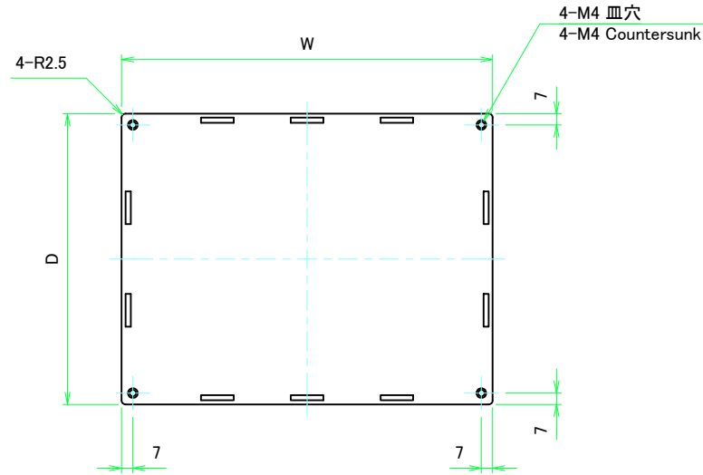
上カバー表面 / Top cover Frontside
