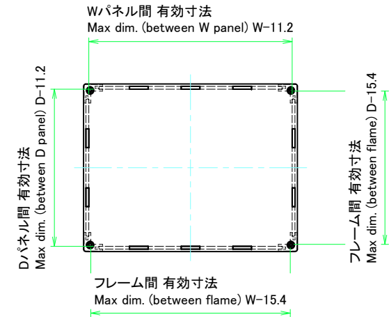
下カバー / Bottom cover
