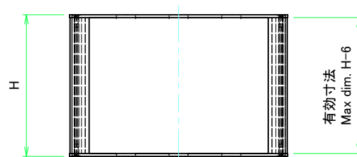
Wパネル1 / W Panel 1
