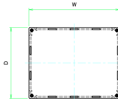
上カバー / Top cover
